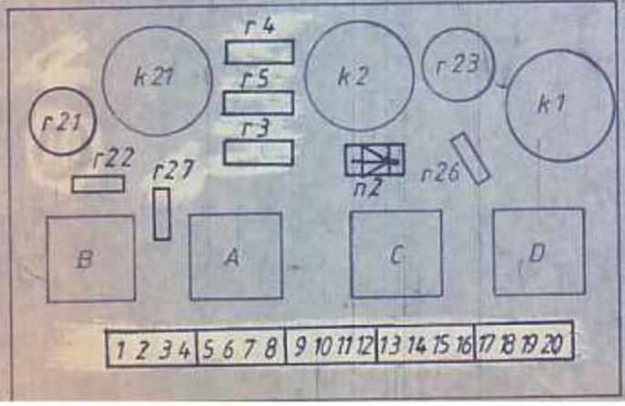
Bestückte Leiterplatte DX 34 Nr. 95-638 549-91
