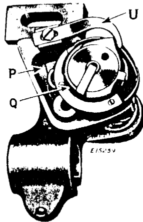
Fig. 6. Hook Lubrication
