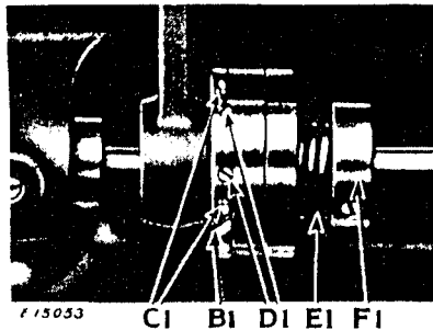
Fig. 24. Feed Eccentric
