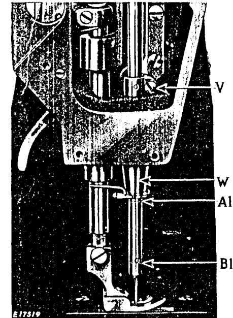
Fig. 24. Setting Needle Bar
