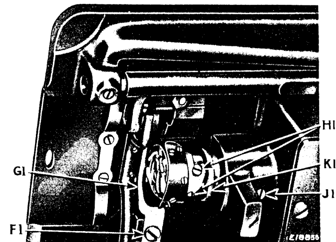
Fig. 25. Removing Hook
