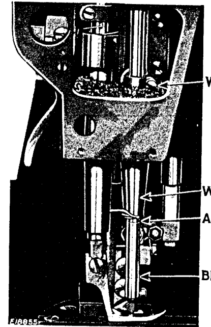
Fig. 23. Setting Needle Bar
