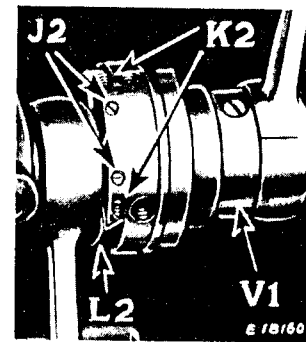
Fig. 29. Feed Eccentric
